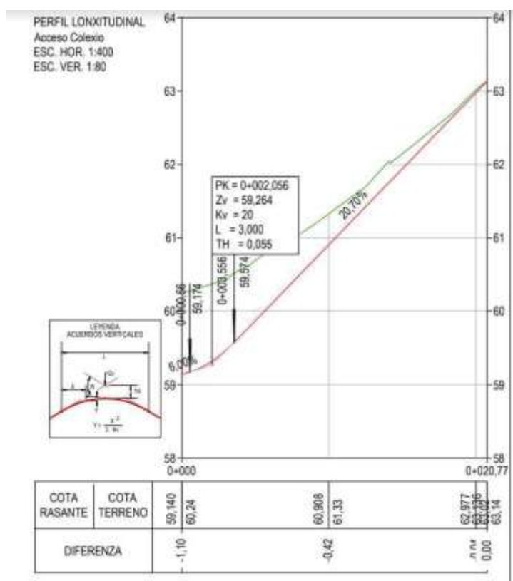
Imaxe 1: Perfil lonxitudinal extraído do proxecto do acceso ao Colexio Milladoiro
