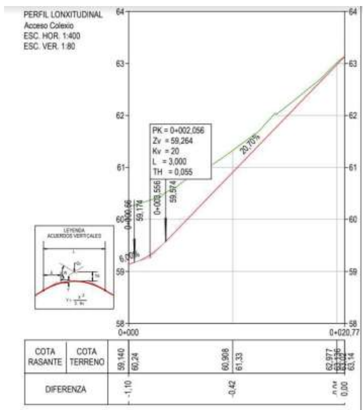
Imaxe 1: Perfil lonxitudinal extraído do proxecto do acceso ao Colexio Milladoiro
